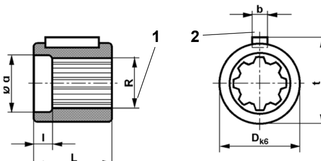
1 Для стандартного шлицевого вала с внешним зацеплением версии «N1» (см. стр. 26) 2 Шпонка согласно DIN 6885
