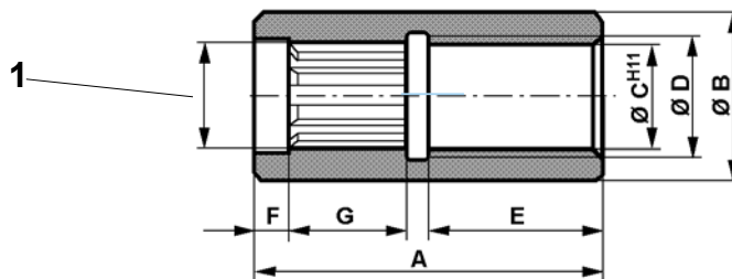
1 Для стандартного шлицевого вала с внешним зацеплением версии «N1» (см. стр. 26)
